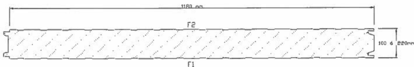
Figure 2 - Section du panneau INDUSTRIAL Agro-alimentaire (IND)
