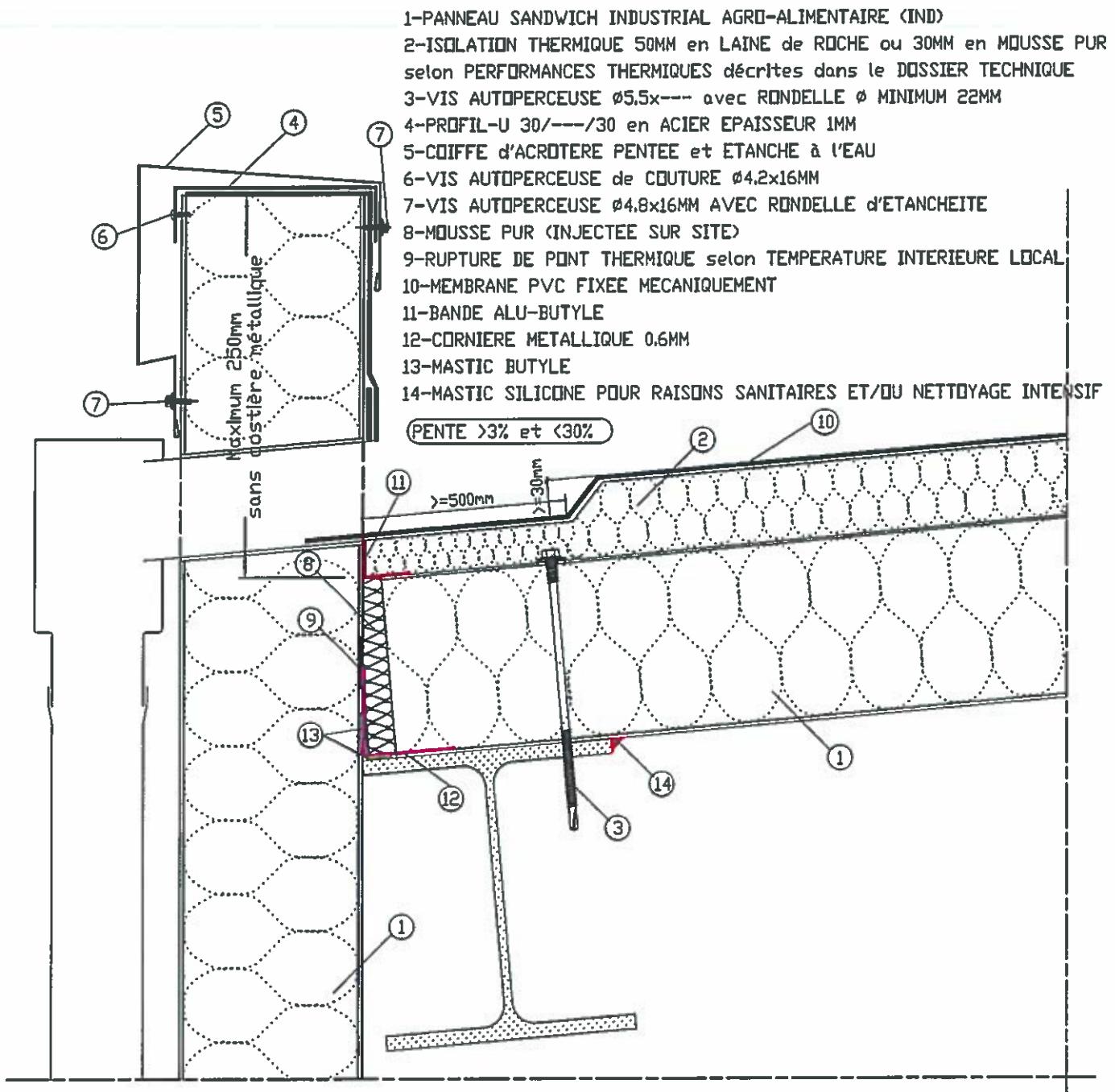
Figure 19 - Bas de pente avec déversoir et boîte à eau gravitaire - hauteur d'acrotère \leq 250 mm Locaux à forte hygrométrie ou pression de vapeur comprise entre 5 et 15 mmHg
