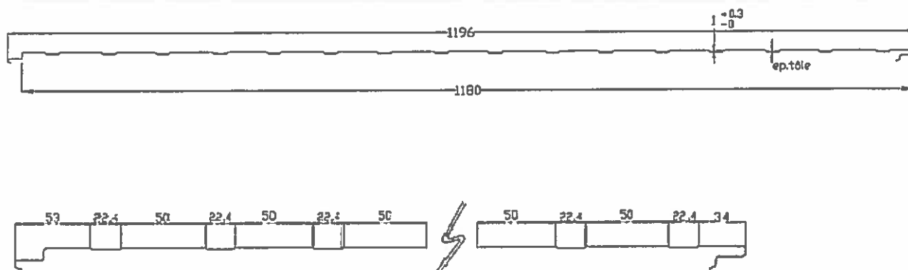
Figure 2 - Section du panneau INDUSTRIAL Agro-alimentaire (IND)
