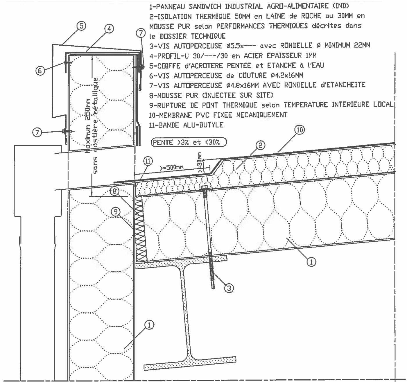
Figure 9 - Bas de pente avec déversoir et boîte à eau gravitaire - Température intérieure local positive Hauteur d'acrotère \leq 250 mm Locaux à faible et moyenne hygrométrie ou pression de vapeur inférieure à 5 mmHg
