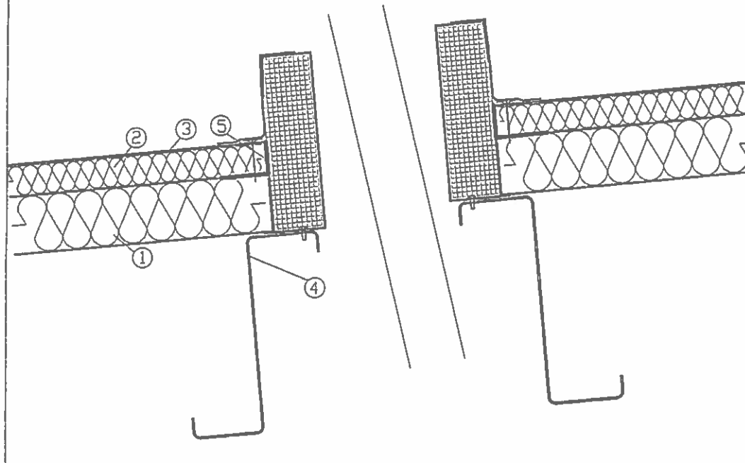
Coupe parallèle à la pente
