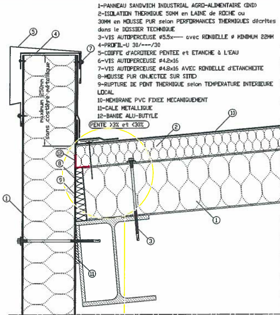
Figure 8 - Bas de pente avec rive en solin - Température Intérieure local positive Hauteur d'acrotère \leq 250 mm Locaux à faible et moyenne hygrométrie ou pression de vapeur inférieure à 5 mmHg
