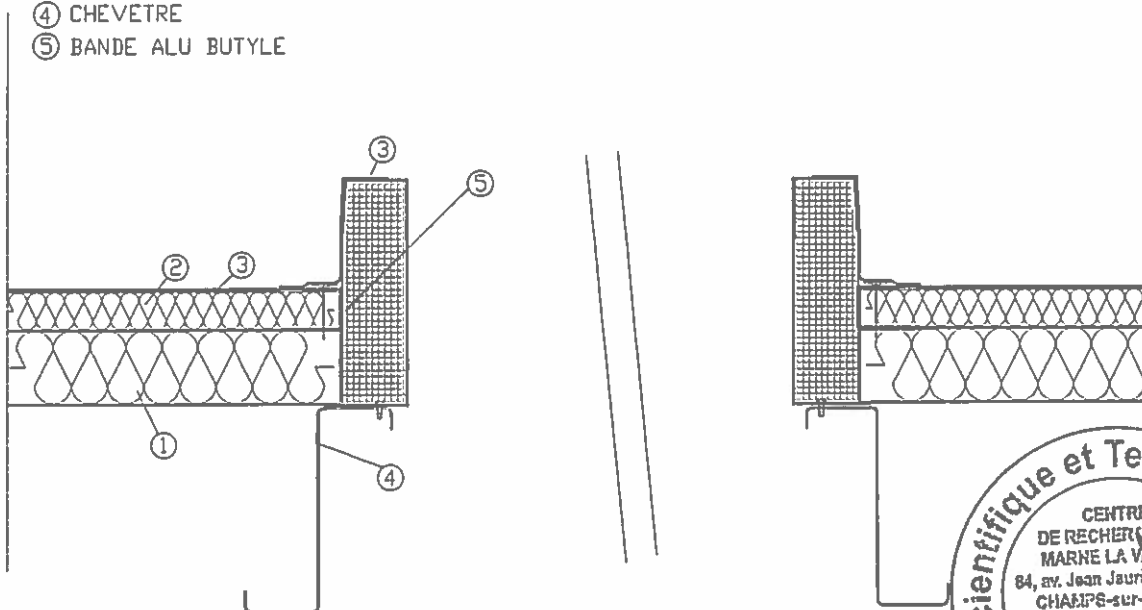
Coupe perpendiculaire à la pente
