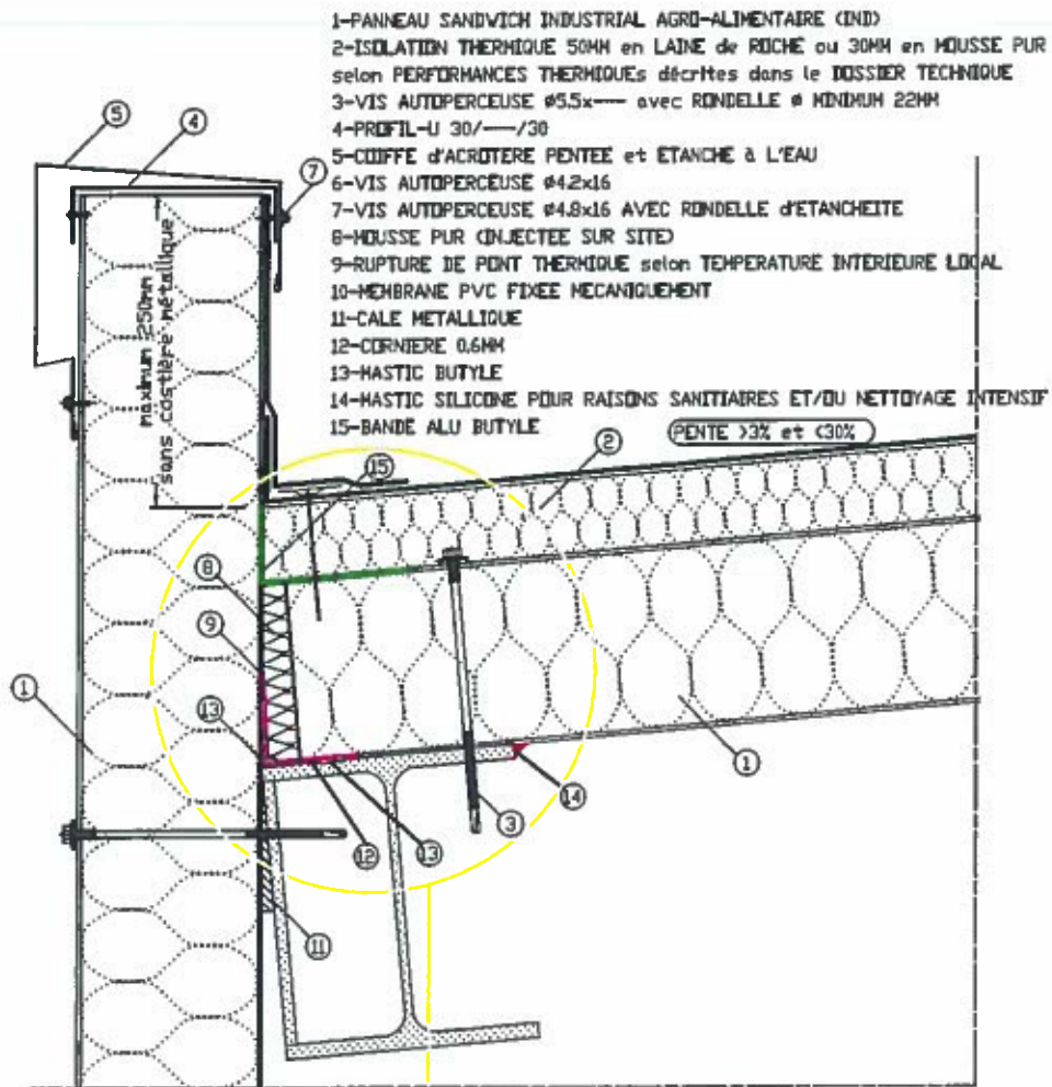
Figure 18 - Bas de pente avec rive en solin - hauteur d'acrotère \leq 250 mm Locaux à forte hygrométrie ou pression de vapeur comprise entre 5 et 15 mmHg
