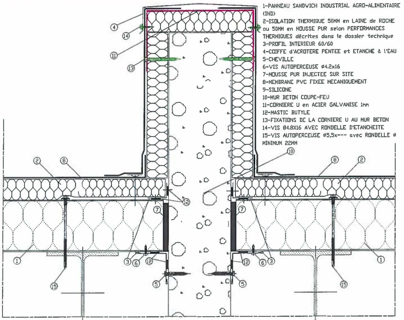
Figure 11 - Dépassement d'une cloison en toiture Locaux à faible et moyenne hygrométrie ou pression de vapeur inférieure à 5 mmHg
