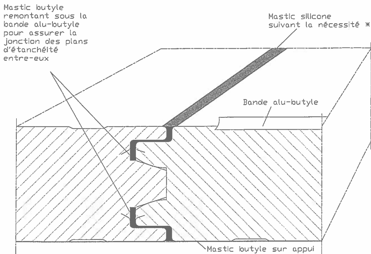
Figure 4 - Croisement des joints Locaux à faible et moyenne hygrométrie ou pression de vapeur inférieure à 5 mmHg
