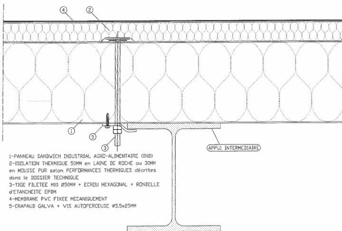
Figure 7 - Jonction sur appui intermédiaire métallique Locaux à faible et moyenne hygrométrie ou pression de vapeur inférieure à 5 mmHg
