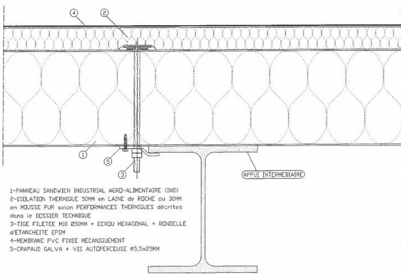
Figure 17 - Jonction sur appui intermédiaire métallique Locaux à forte hygrométrie ou pression de vapeur comprise entre 5 et 15 mmHg
